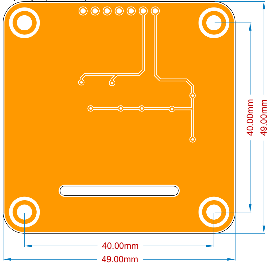
Top Layer (Scale 2:1)
