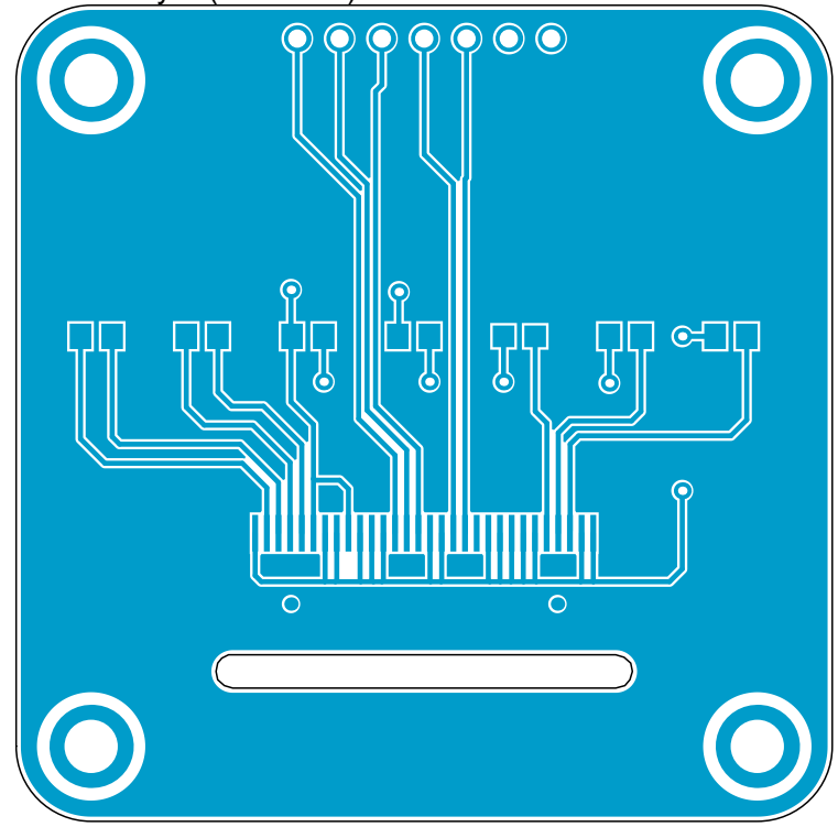
Bottom Layer (Scale 2:1)
