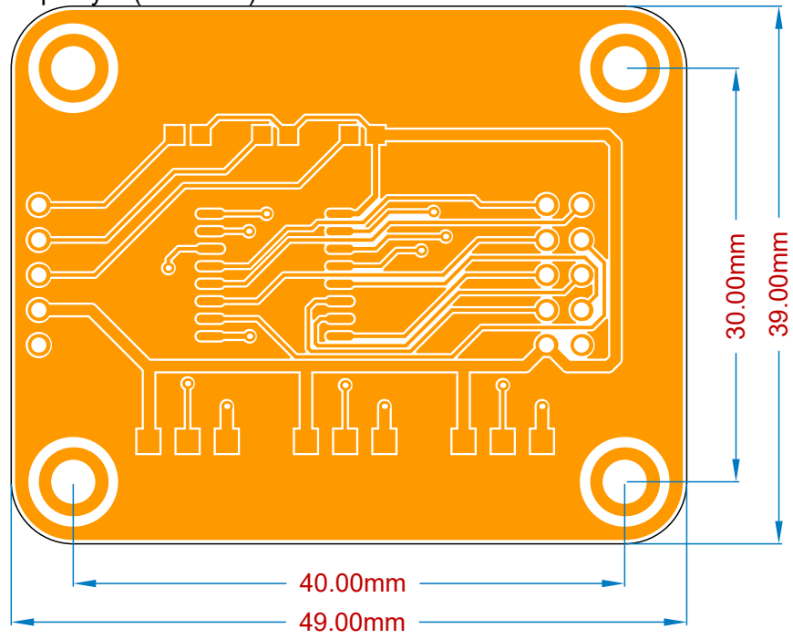
Top Layer (Scale 2:1)
