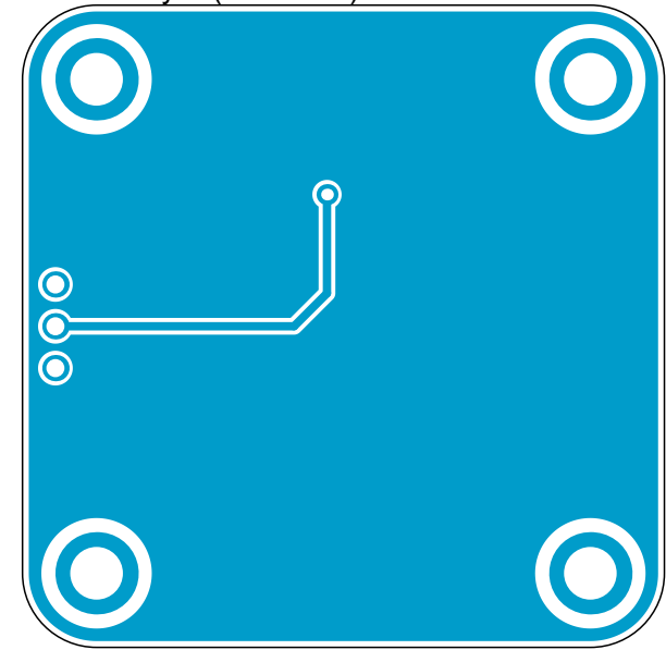
Bottom Layer (Scale 2:1)
