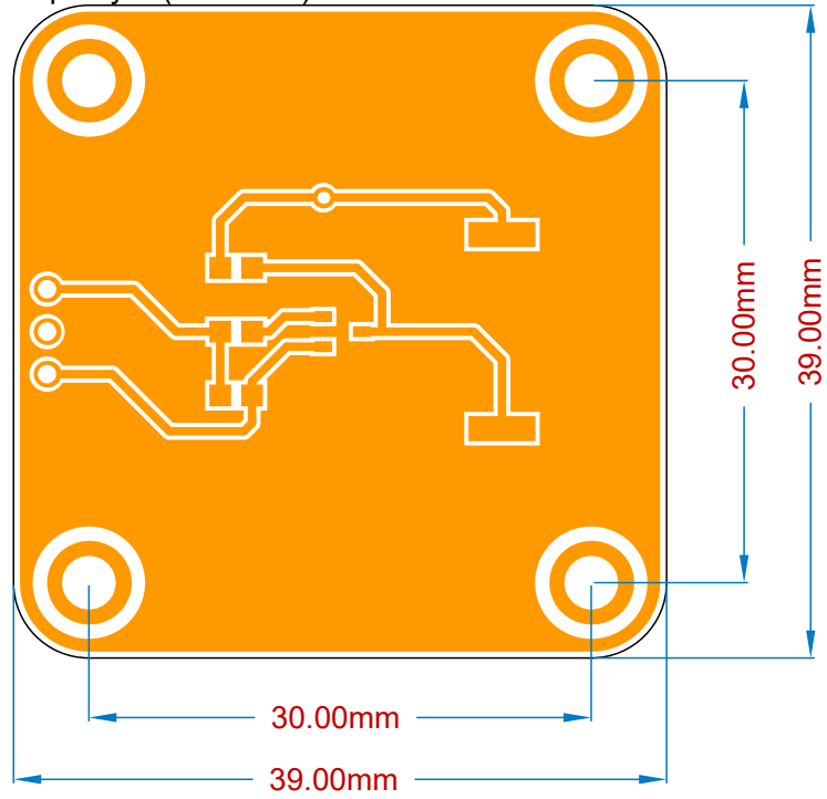
Top Layer (Scale 2:1)
