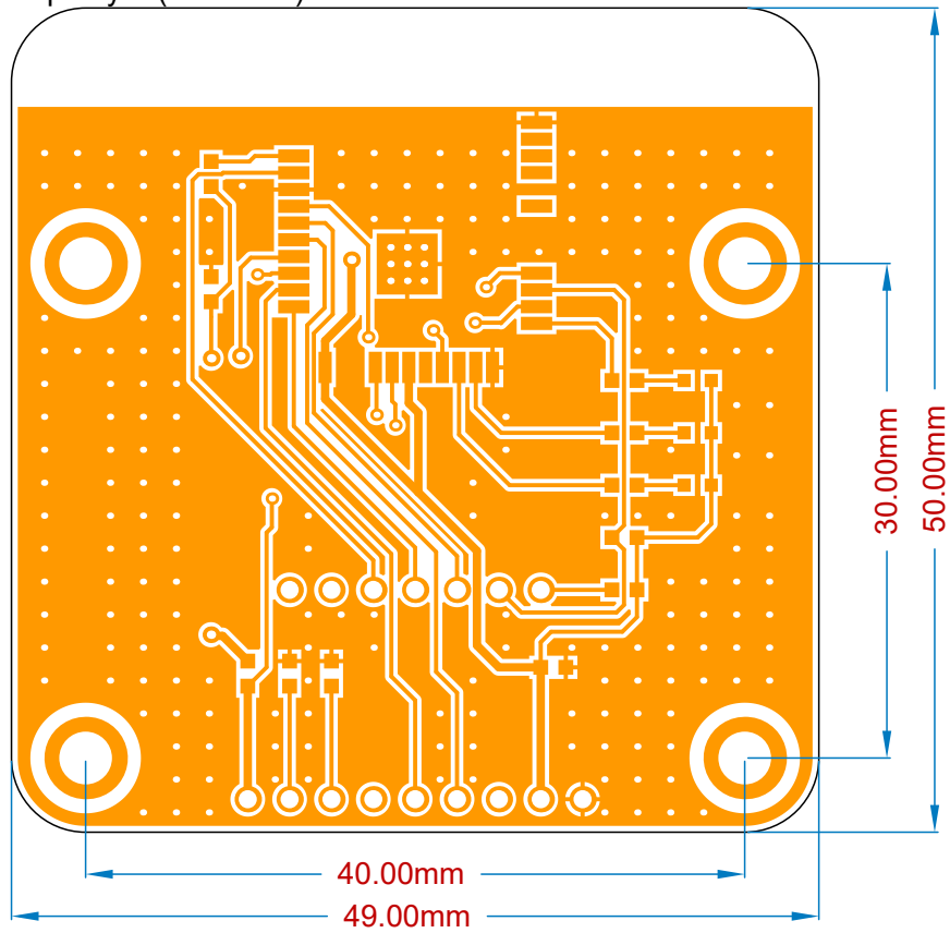
Top Layer (Scale 2:1)
