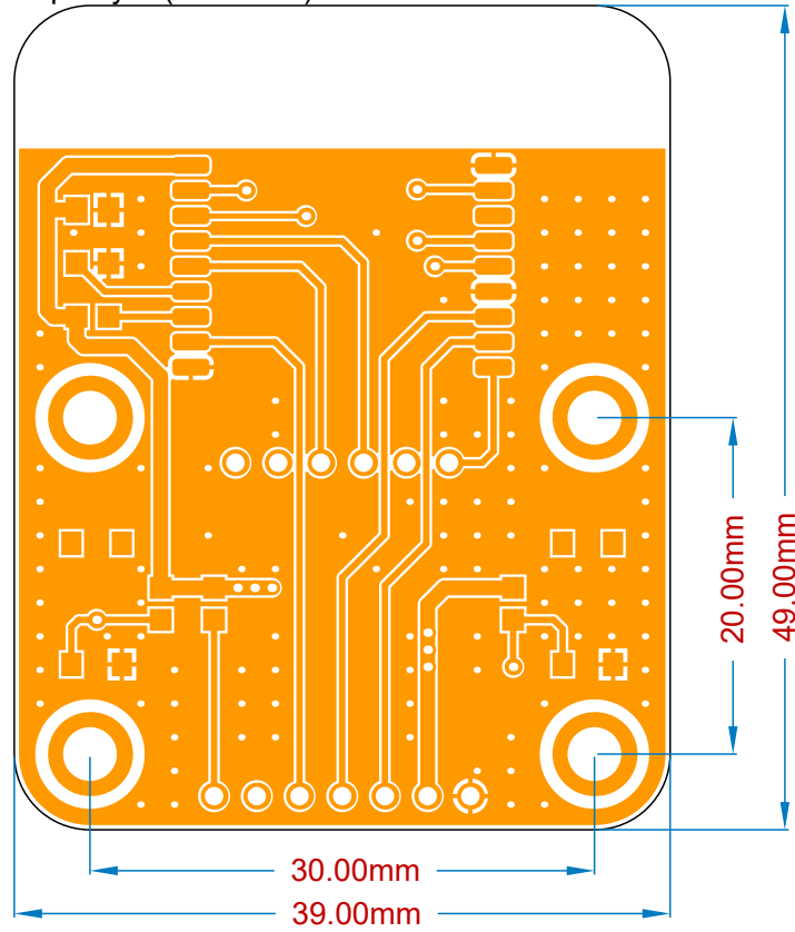
Top Layer (Scale 2:1)
