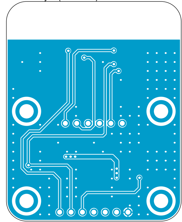
Bottom Layer (Scale 2:1)
