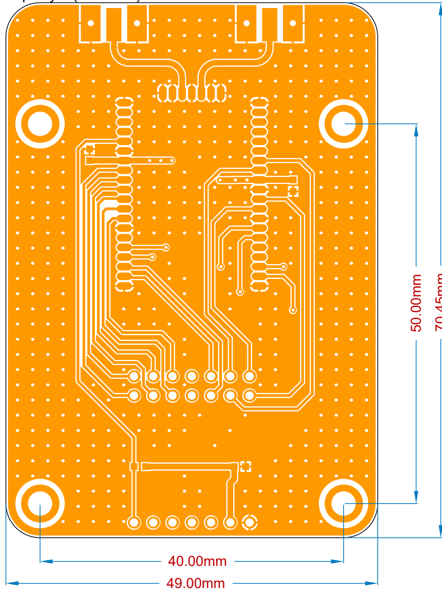
Top Layer (Scale 2:1)
