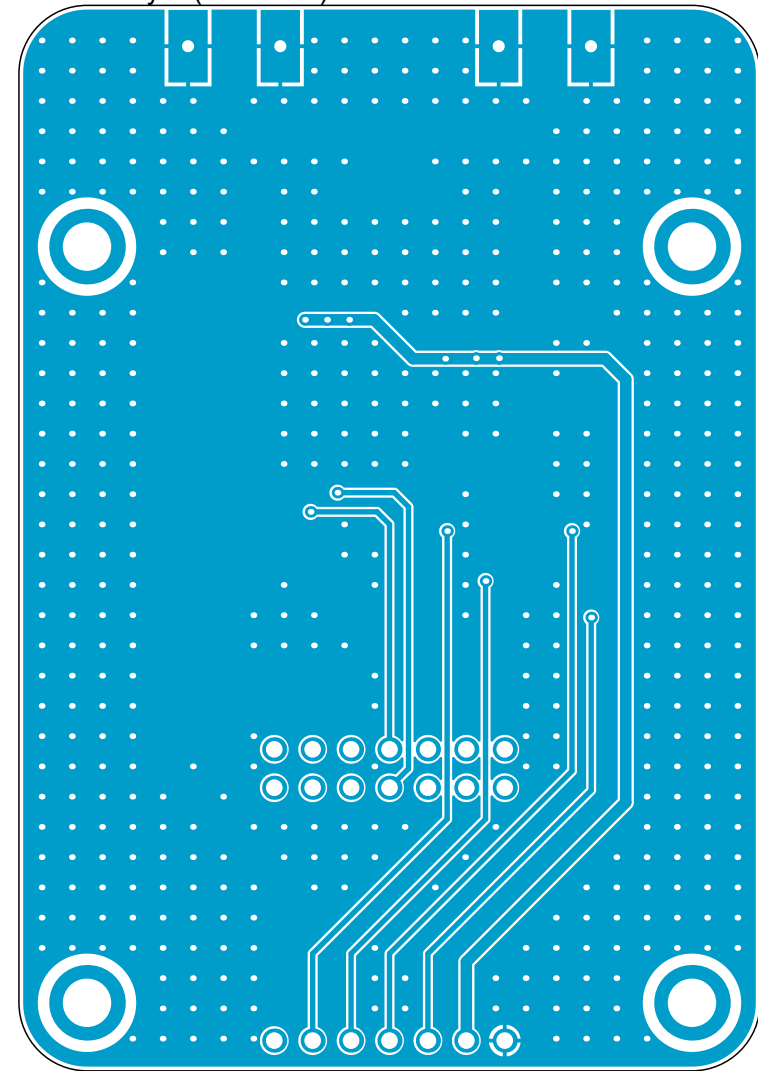
Bottom Layer (Scale 2:1)
